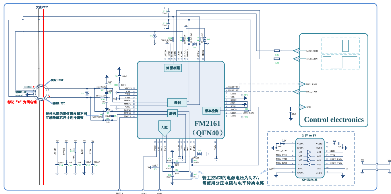
图 5-1 FM2161A 的典型应用电路图
