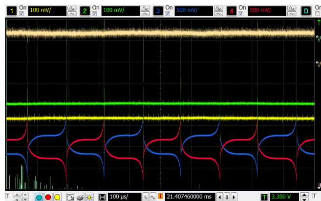
(1-2 通道为差分解调输出，3-4 通道为调制输入，f1=2 通道-1 通道)
